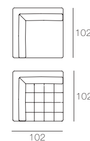
Divano letto_Sofa bed
