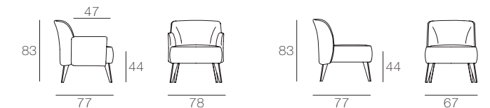
CON PIEDINI - WITH FEET
